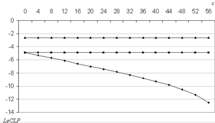
Рисунок 1 – Залежність ймовірностей втрат різнотипних заявок від параметра за B = 60 : \lambda_1 = 0,1 ; \lambda_2 = 0,85 ; \blacktriangle – CLP_i ; \blacksquare – CLP_2 ; \blacklozenge – CLP_1
