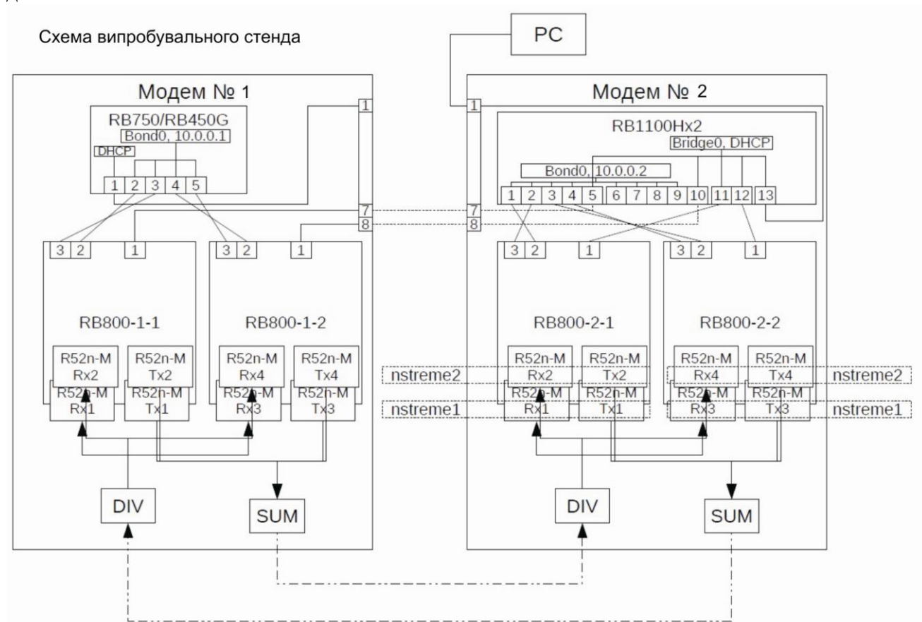
Рисунок 3- Структурна схема випробувального стенда
