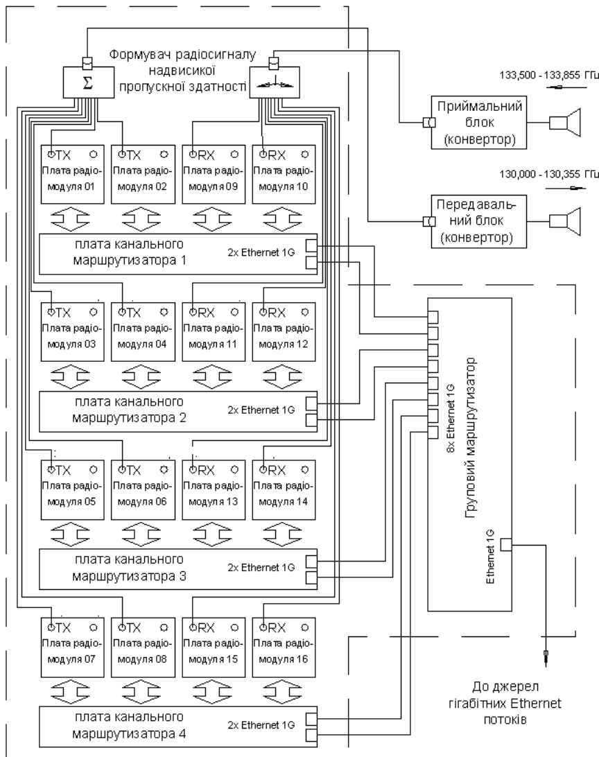
Рисунок 1 – Структурна схема модема надвисокої (2,4 Гбіт/с) пропускної здатності
