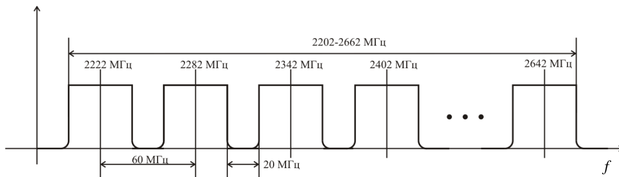
Рисунок 2 – Частотний план модема
