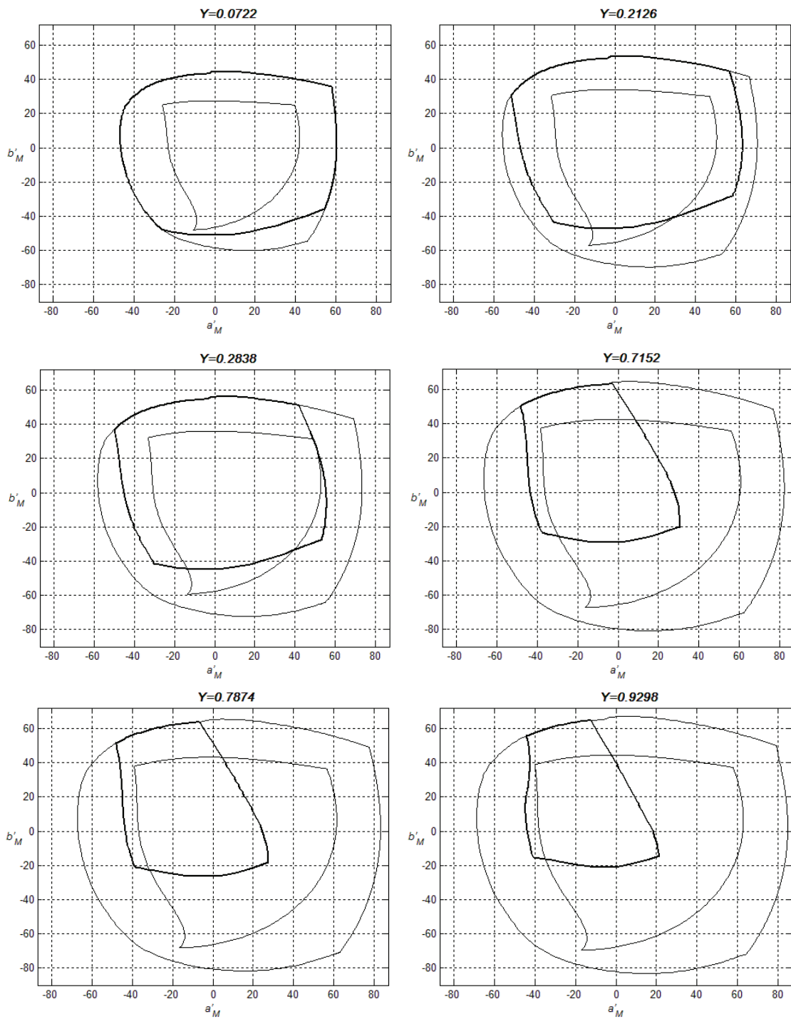
Рисунок 22 – Розширена область передаваних кольорів в координатах (a'_M, b'_M) у системі телебачення високої чіткості для яскравості адаптації L_A = 200 \text{ кд/м}^2 й середнього оточення
