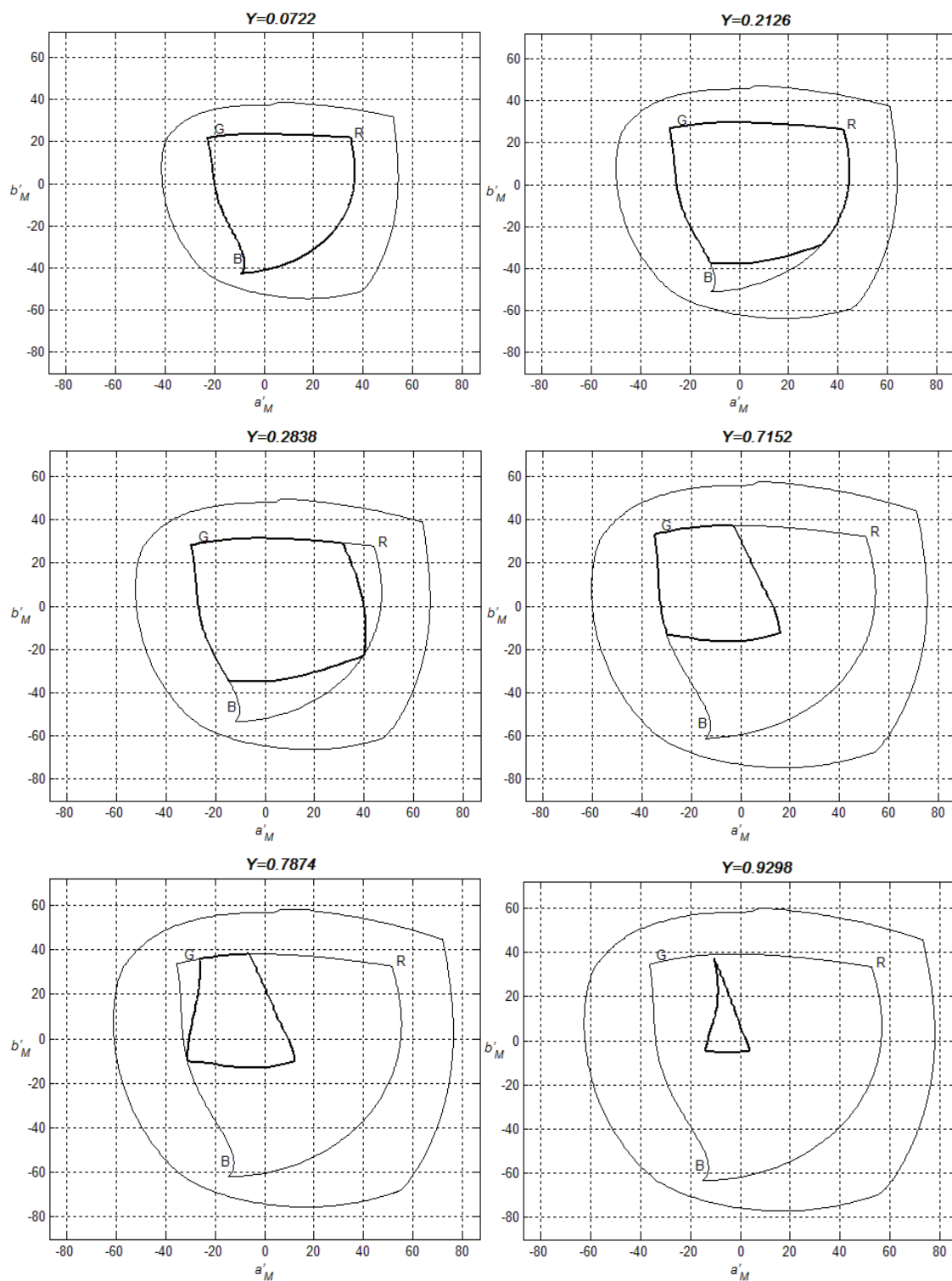
Рисунок 9 – Область кольорів у просторі SAM02-UCS ( a'_M, b'_M ), передаваних системами ТБВЧ, для яскравості адаптації L_A = 20 кд/м 2
