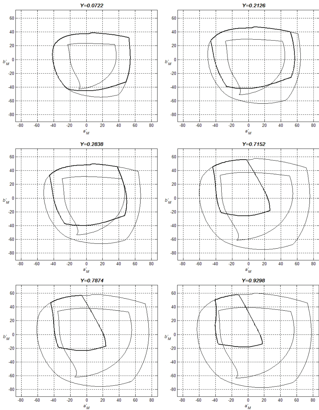
Рисунок 21 – Розширена область передаваних кольорів в координатах (a'_M, b'_M) у системі телебачення високої чіткості для яскравості адаптації L_A = 20 кд/м 2 й середнього оточення
