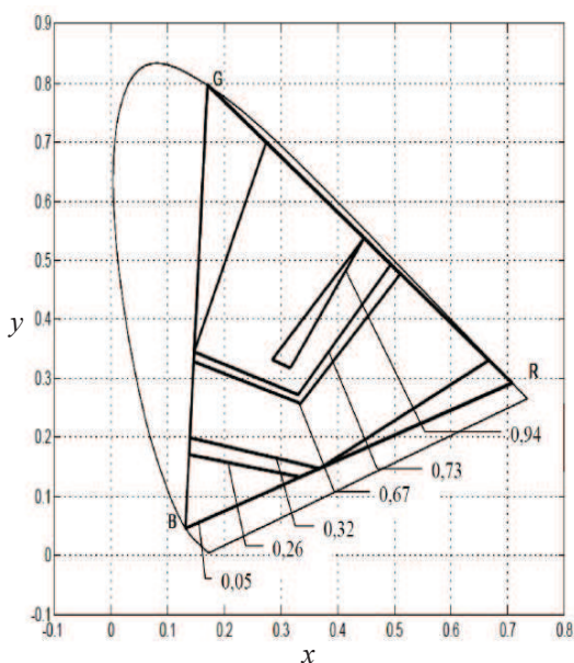
Рисунок 3 – Область кольорів, передаваних системами ТБНВЧ
