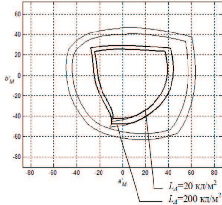
Рисунок 21 – Вплив яскравості адаптації на область кольорів, передаваних у системі ТБВЧ, для яскравості стимулу Y = 0,1
