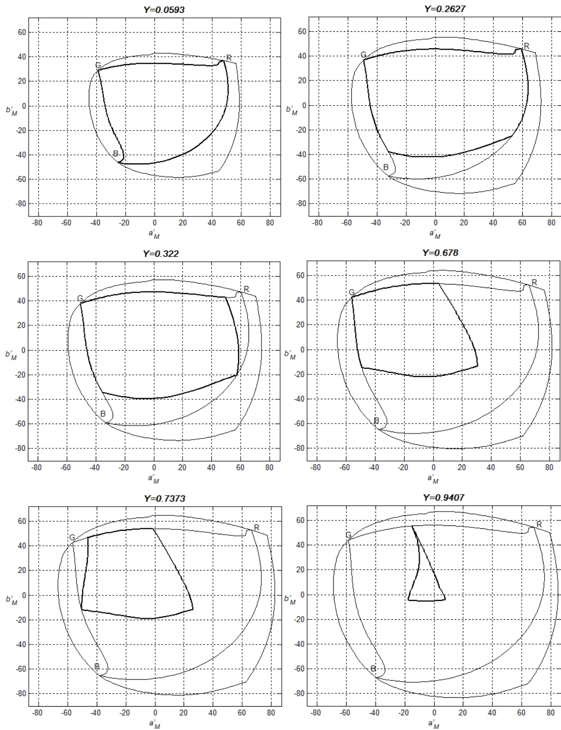
Рисунок 12 – Область кольорів у просторі SAM02-UCS ( a'_M, b'_M ), передаваних системами ТБНВЧ, для яскравості адаптації L_A = 200 кд/м 2
