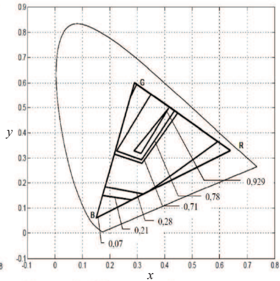
Рисунок 2 – Область кольорів, передаваних системами ТБВЧ
