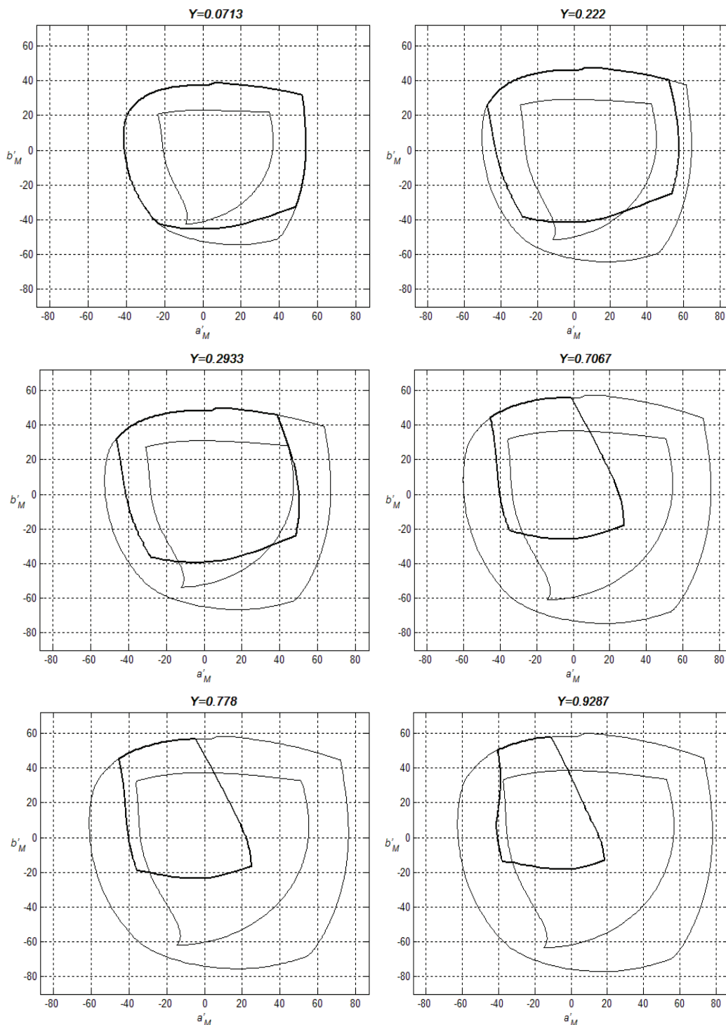
Рисунок 19 – Розширена область кольорів, передаваних у системі ТБСЧ, в координатах ( a'_M, b'_M ) для яскравості адаптації L_A = 20 кд/м 2 й середнього оточення.
