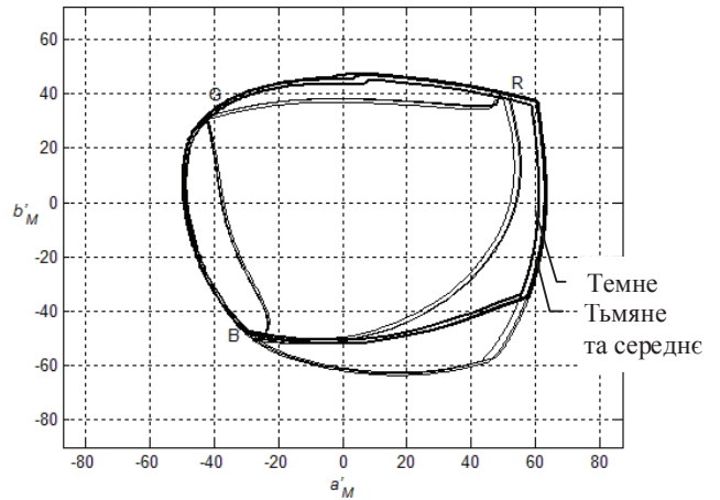
Рисунок 28 – Вплив яскравості адаптації на область кольорів, передаваних у системі ТБВЧ, для яскравості стимулу Y = 0,25
