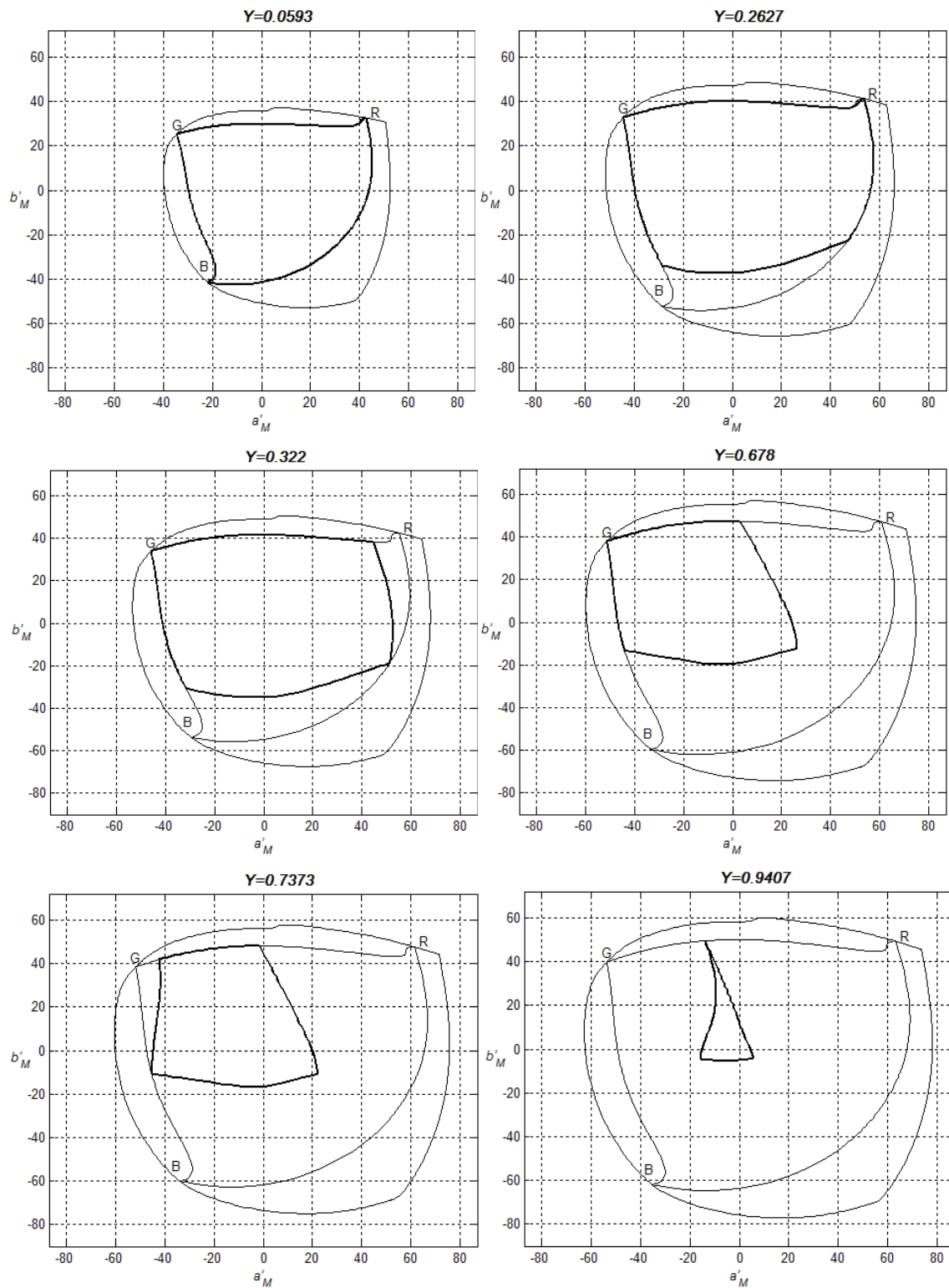
Рисунок 11 – Область кольорів у просторі CAM02-UCS ( a'_M, b'_M ), передаваних системами ТБНВЧ, для яскравості адаптації L_A = 20 \text{ кд/м}^2
