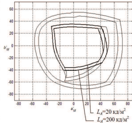
Рисунок 22 – Вплив яскравості адаптації на область кольорів, передаваних у системі ТБВЧ, для яскравості стимулу Y = 0,25
