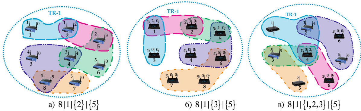
Рисунок 12 – Пример решения задачи распределения четырех ЧК в mesh-сетях с различным числом РИ на станциях и числом неперекрывающихся ЧК, не превышающим число станций
