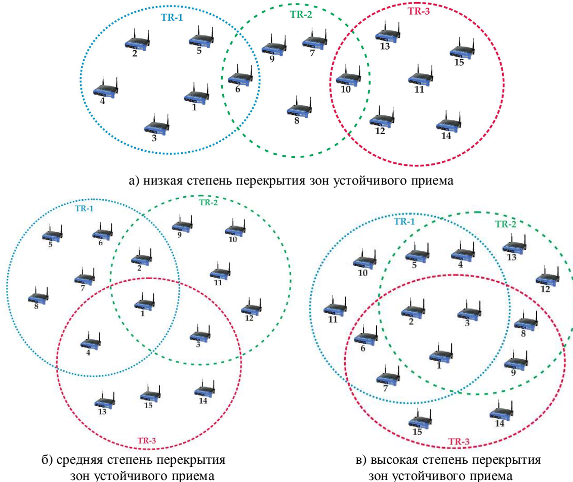
Рисунок 7 – Пример возможных конфигураций mesh-сетей 15|3|\{2\}|\{4\} с различной степенью перекрытия зон устойчивого приема
