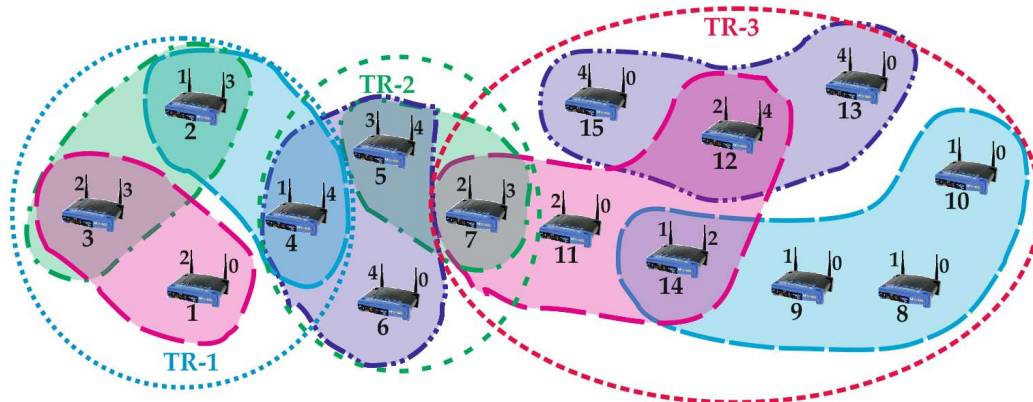
Рисунок 10 – Пример решения задачи распределения четырех ЧК для mesh-сети 15|3|\{2\}|\{4\} с неоднородными зонами устойчивого приема
