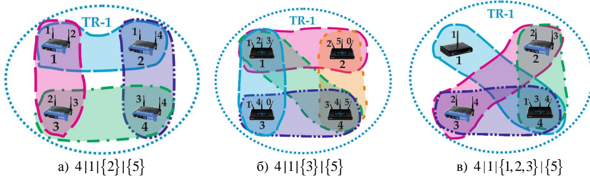
Рисунок 14 – Пример решения задачи распределения четырех ЧК в mesh-сетях с различным числом РИ на станциях и числом неперекрывающихся ЧКЖ, превышающим число станций
