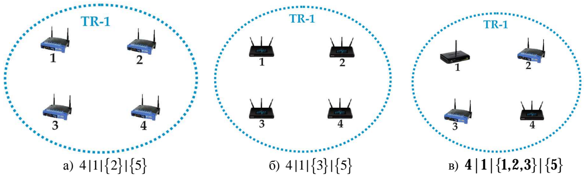
Рисунок 13 – Примеры возможных конфигураций mesh-сетей с различным числом РИ на станциях и числом неперекрывающихся ЧК, превышающим число станций
