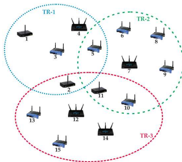
Рисунок 2 – Пример mesh-сети с указанием зон устойчивого приема при Z = 3 и N = 15 Mesh-сети, приведенной на рис. 1, соответствует следующая TR-матрица:
