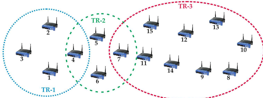
Рисунок 9 – Пример возможной конфигурации mesh-сети 15|3|\{2\}|\{4\} с различными размерами зон устойчивого приема
