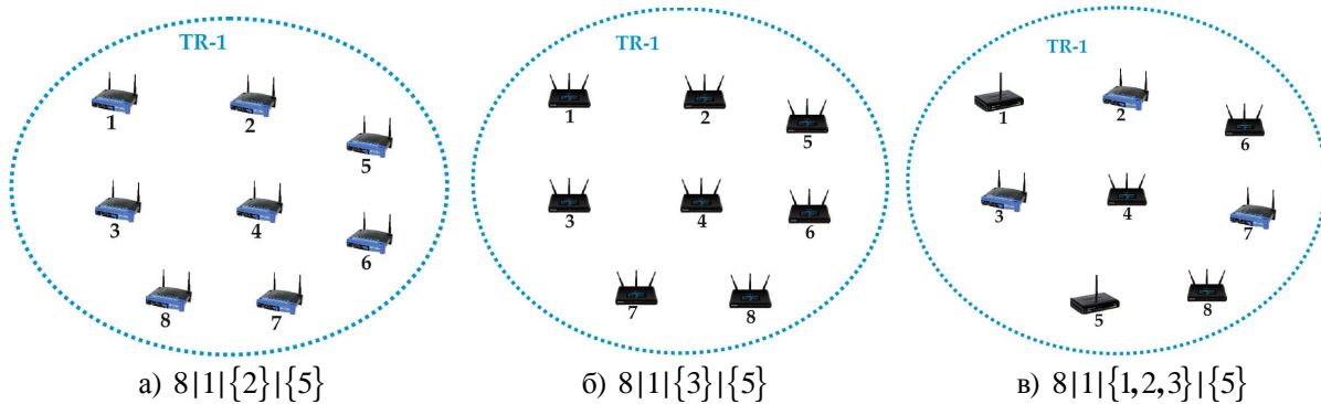
Рисунок 11 – Примеры возможных конфигураций mesh-сетей с числом станций, превышающим число используемых неперекрывающихся ЧК
