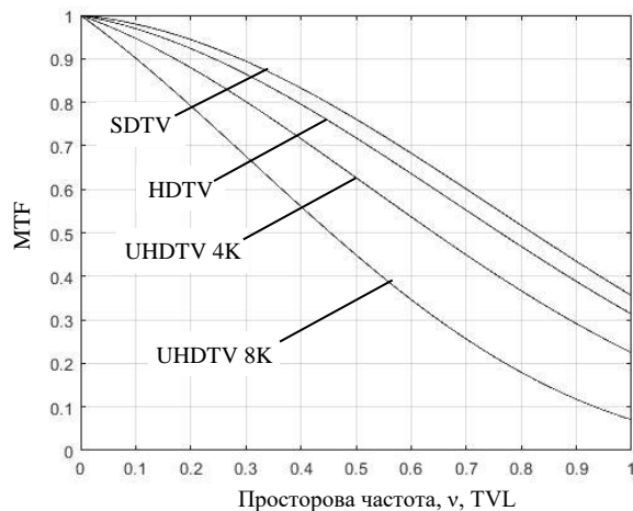
Рисунок 10 – Просторова КЧХ ідеального ТВ тракту «від світла до світла» для D/f=1:6 , h_s=10 мм
